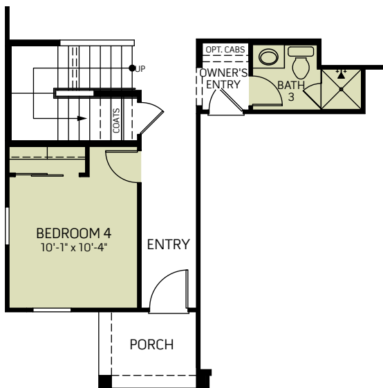
OPTIONAL BEDROOM 4/BATH 3 ILO DEN
